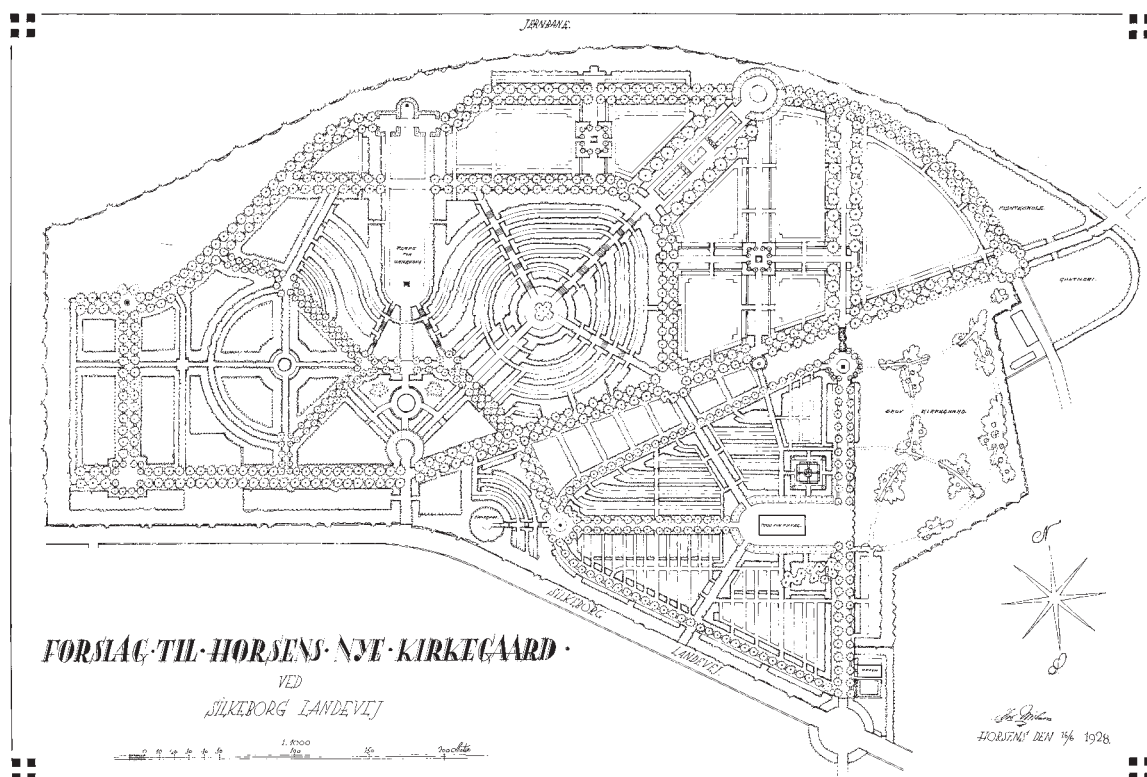
Fig. 13. Vestre Kirkegård. Forslag til kirkegårdens anlæg ved Chr. Nielsen 1928 (s. 6132). Kun det sydøstre afsnit blev udført efter planen. Tegning i kirkegårdskontoret. 1:5000. – Vestre Kirkegård. Proposal for the layout of the cemetery by Chr. Nielsen, 1928. Only the southeastern section was executed according to the plan.
