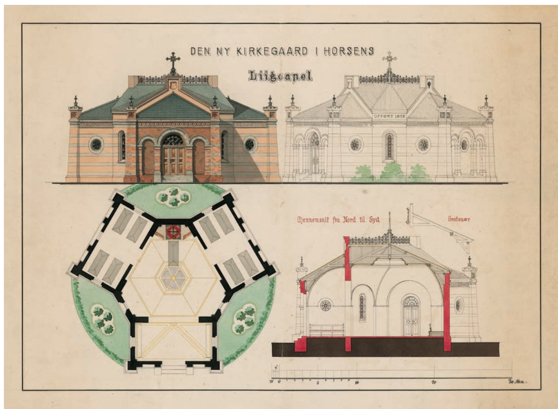
Fig. 10. Projekt til ligkapel ved Jens Chr. Clausen 1875 (s. 6128). Tegning i Horsens Museum. 1:300. — Project for mortuary chapel by Jens Chr. Clausen, 1875.
