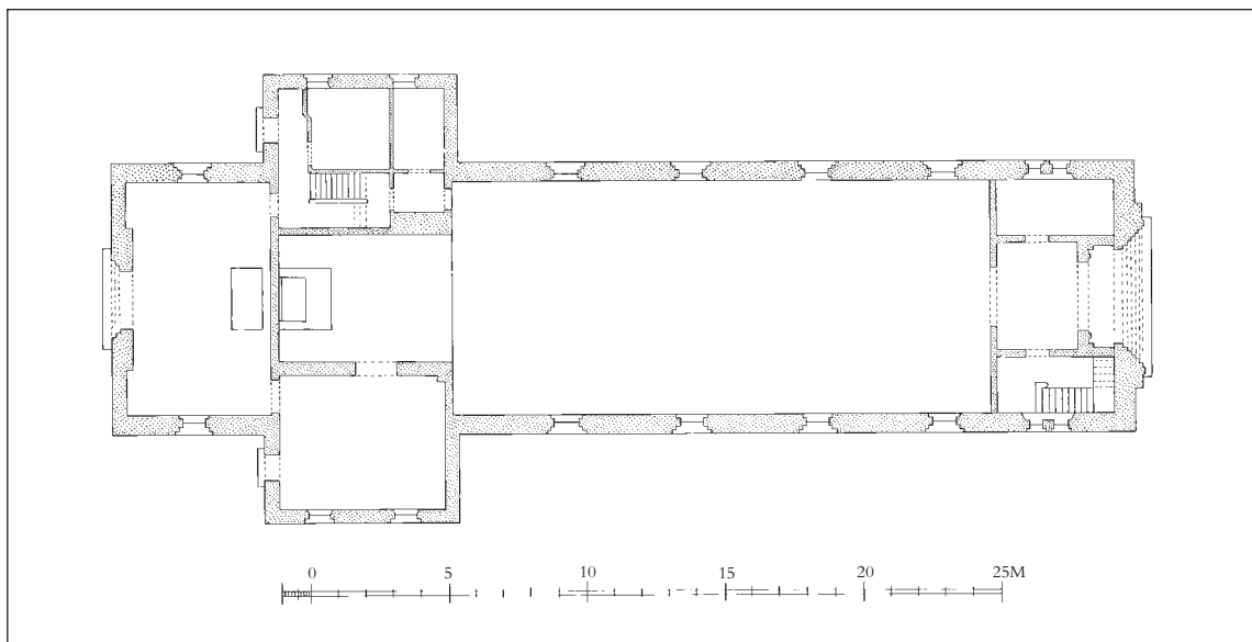
Fig. 15. Grundplan 1:300 af kapel med krematorium, opført 1938 ved Viggo Norn (s. 6133). Tegnet af Marianne Nielsen 2004 efter plan 1947 i Horsens Museum. – Ground plan 1:300 of chapel with crematorium, built in 1938, by Viggo Norn.
