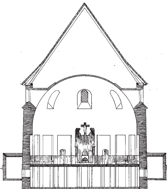
TVÆRSNIT
